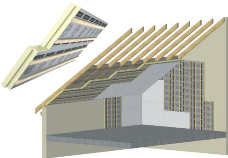
Neben der kurzen Montagezeit bietet die neue Innendämmung LINITHERM PAL UK eine minimale Aufbauhöhe dank hoher Dämmeffizienz (λ 0,023). Die raumseitige Beplankung ist frei wählbar, die elektrische Ausstattung (LED-Spots, Steckdosen etc.) lässt sich schnell und sicher einbauen oder nachrüsten.
